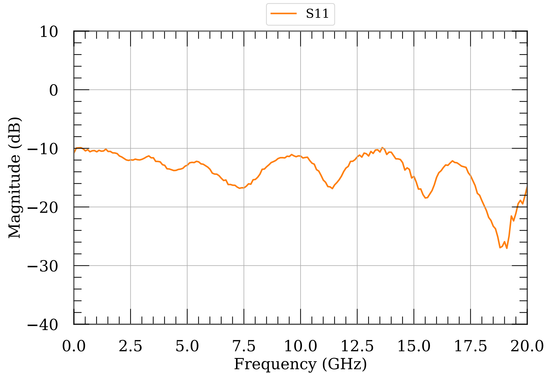
LNA S-params module006
